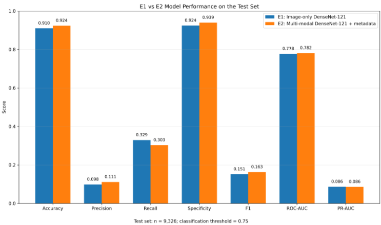
Figure 3.5.1: E1 and E2 comparison.
